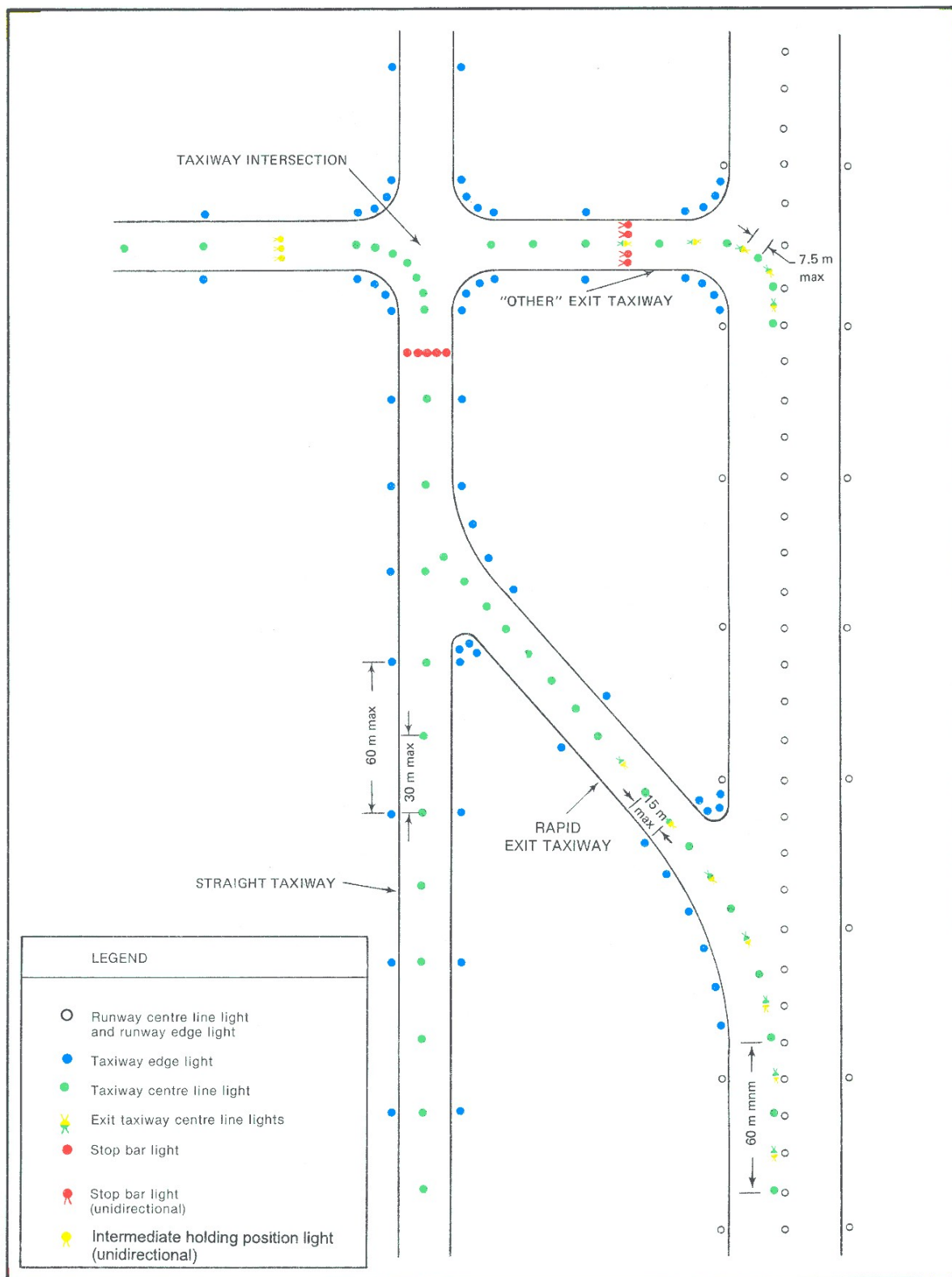
Figura 20 – Immagine riassuntiva luci di pista e taxiway
