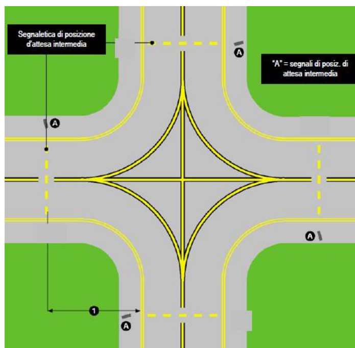
Figura 16 – Segnaletica orizzontale Intermediate Holding Position (IHP)
