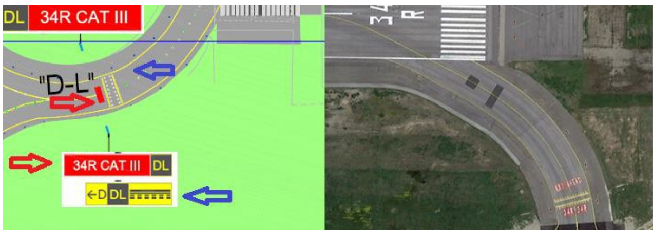
Figura 13 – Esempio di segnaletica di obbligo su TWY DL
