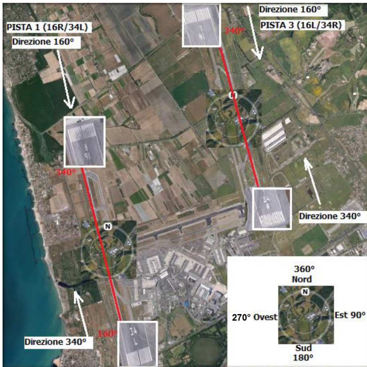
Figura 2 – Piste 16R/34L e 16L/34R
